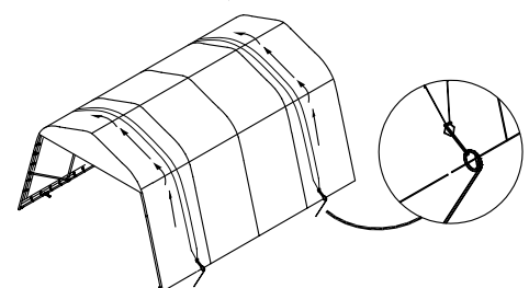
FIG. I BANDE ANTI-VENT / WINDSECURE KIT OPTIONNEL / OPTIONAL
